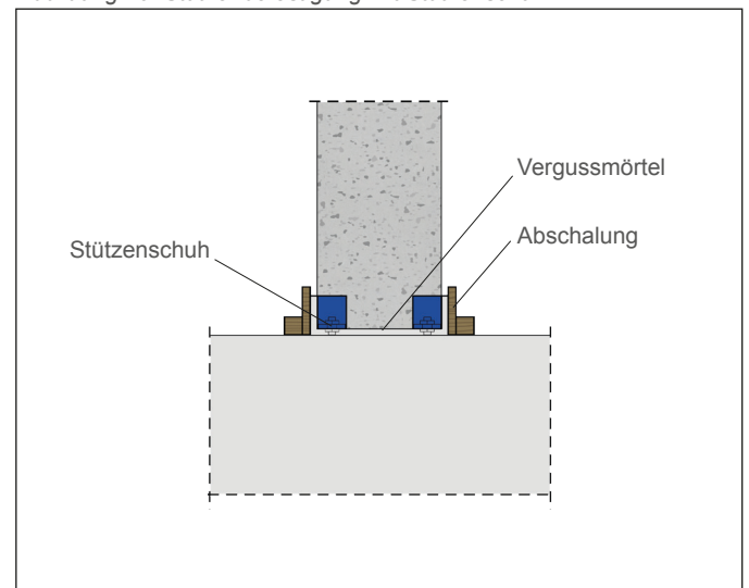
Abbildung 10: Stützenbefestigung mit Stützenschuh
