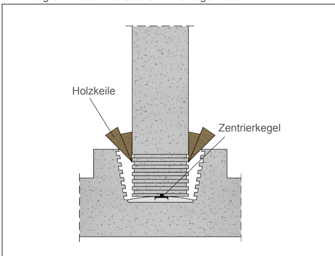
Abbildung 8: Fixieren der Stütze im Montagezustand
