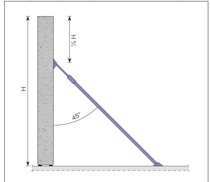
Abbildung 3: Montagesicherung einer Massivwand mit Schrägstützen
