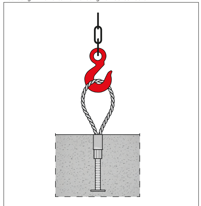
Abbildung 1: Korrekte Verwendung von Seilschlaufen
