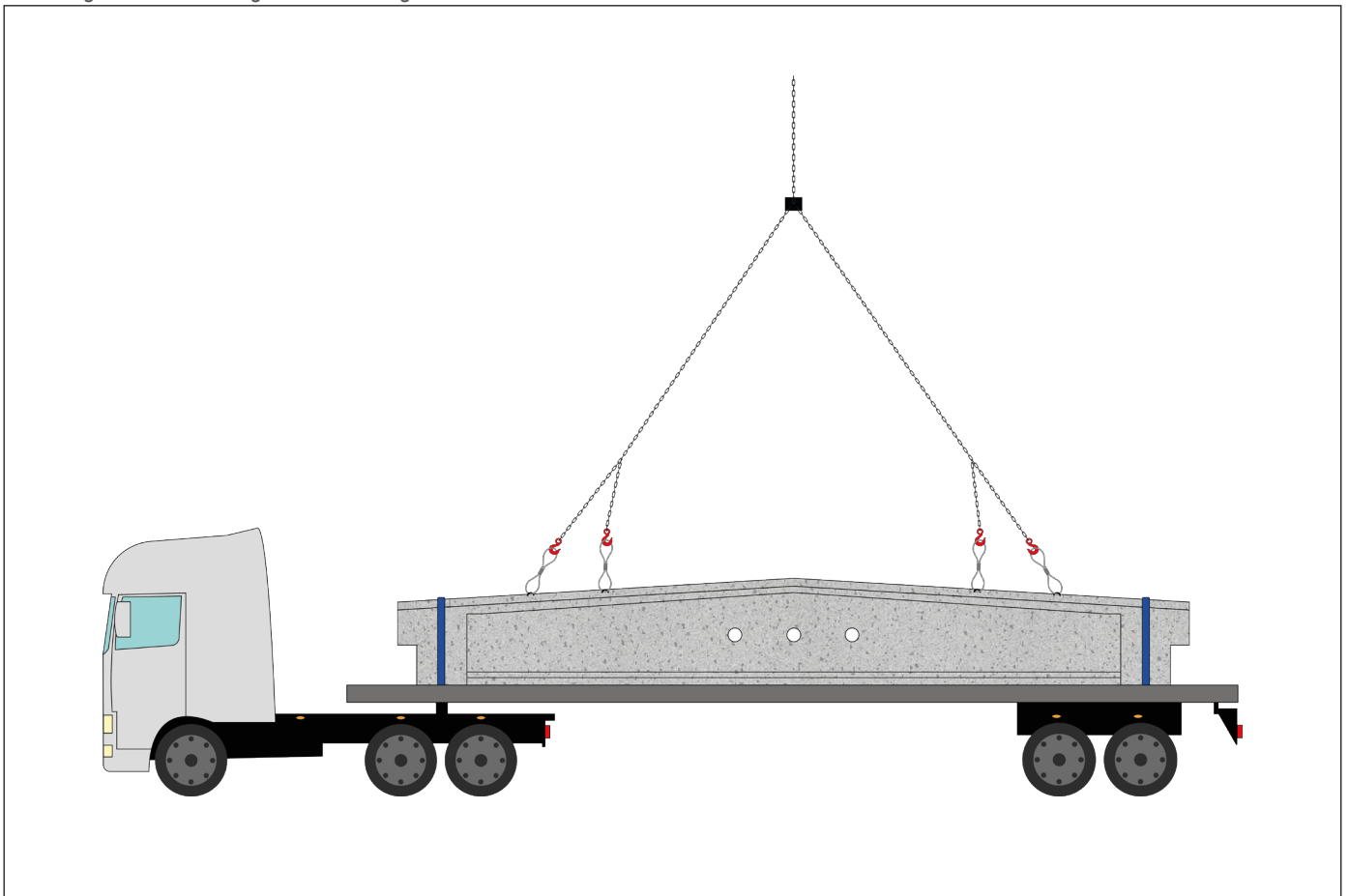
Abbildung 11: Bindermontage vom Fahrzeug
