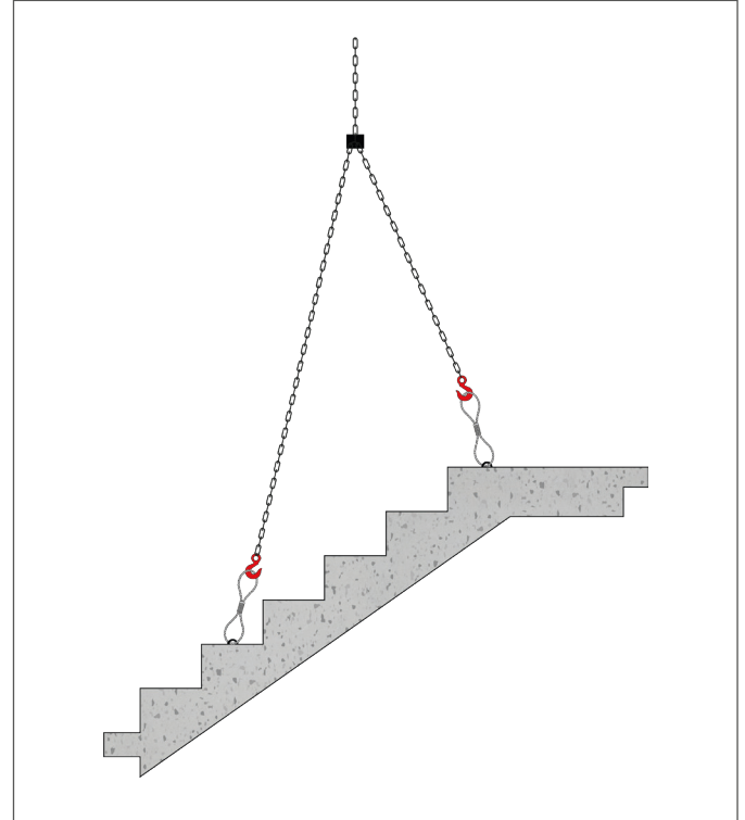
Abbildung 6: Korrektes Ausrichten des Treppenlaufes vor der Montage
