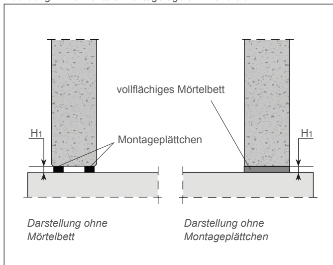
Abbildung 2: Horizontale Montagefuge am Wandfuß
