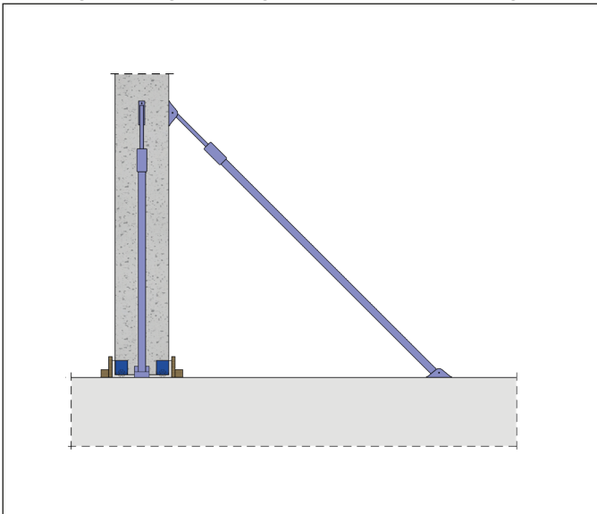
Abbildung 9: Montagesicherung einer Stütze mit 2 Druck-Zugstreben
