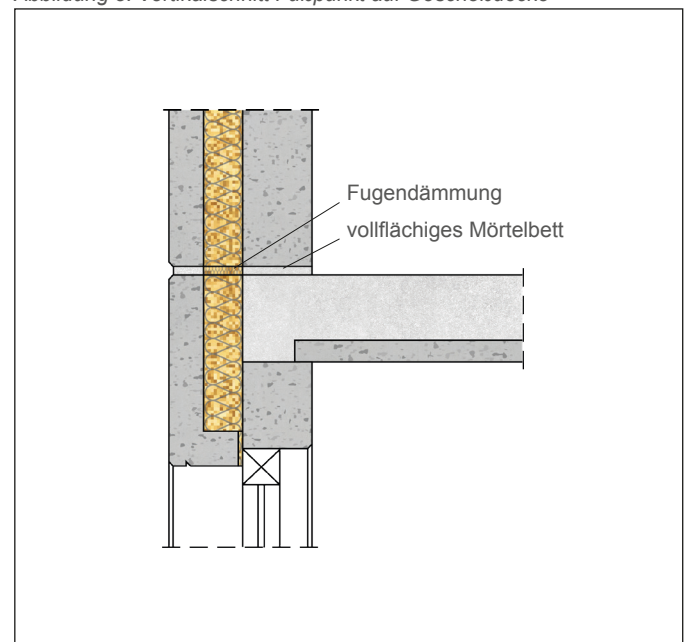
Abbildung 5: Vertikalschnitt Fußpunkt auf Geschoßdecke
