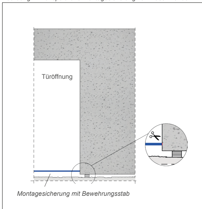
Abbildung 4: Transport- und Montagesicherung von Massivwänden
