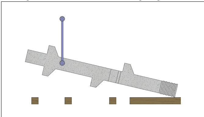
Abbildung 7: Aufrichten einer Stütze mit Stützensgehänge
