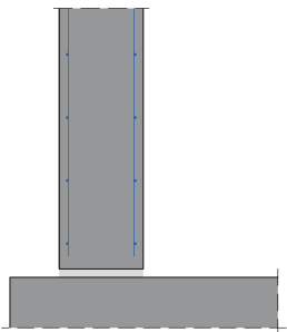
Wandanschluss Bodenplatte Außenwand ohne Gleitsicherung
