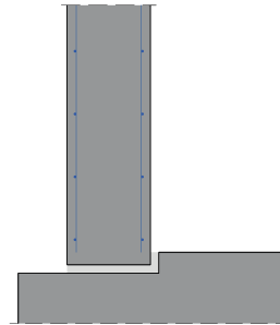
Wandanschluss Bodenplatte Außenwand mit Gleitsicherung, Bodenplatte mit Versatz
