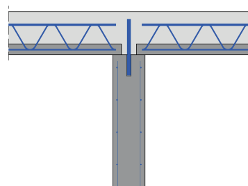
Deckenanschluss, tragende Innenwand mit Dorn am Wandkopf, mit Elementdecke
