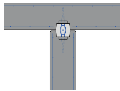
Wandstoß T-Form durchlaufende Wand mit Vergussnut und Seilschlaufe
