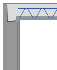
Deckenanschluss Außenwand mit Randaufkantung und Nut am Wandkopf, mit Elementdecke
