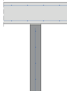
Deckenanschluss Außenwand mit Randaufkantung und Nut am Wandkopf, mit Elementdecke
