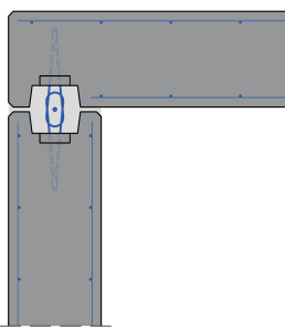
Wandanschluss Bodenplatte Außenwand ohne Gleitsicherung
