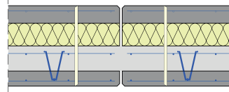
Wandstoß gerade mit Schöck Isolink®
