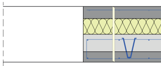
Wand Fensteröffnung mit Schöck Isolink®
