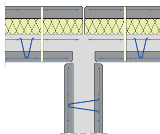
Wandstoß T-Form mit Schöck Isolink®
