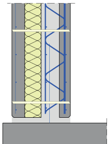
Wandanschluss Bodenplatte mit Schöck Isolink® Anschlussbewehrung mittig
