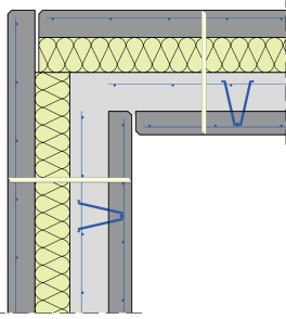
Wandstoß Ecke mit Schöck Isolink®
