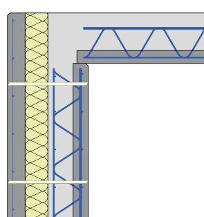
Deckenanschluss mit Schöck Isolink® schematisch
